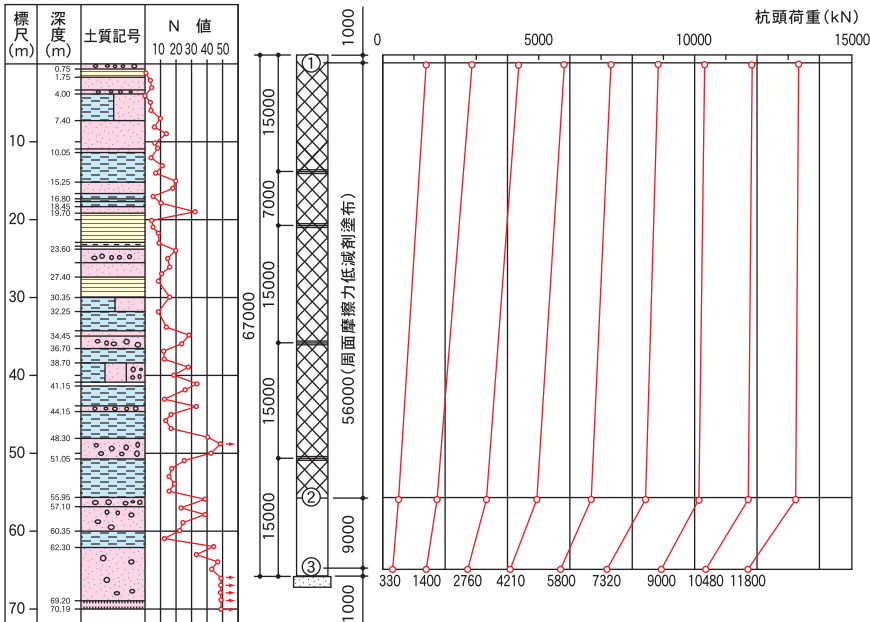
軸力分布図
