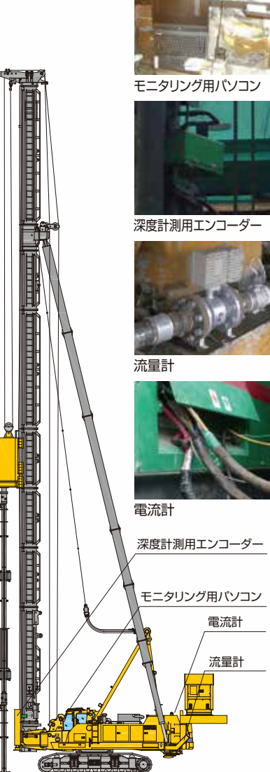
施工管理装置 取付例
