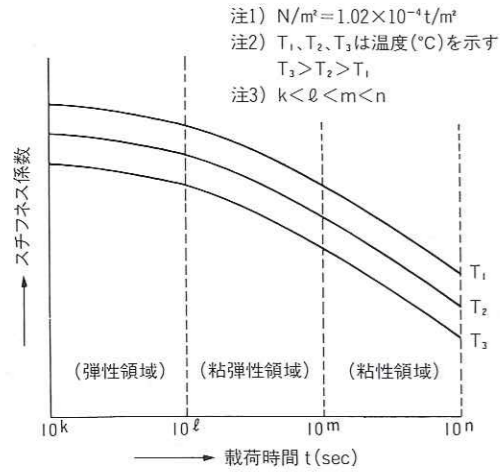
スチフネス係数と荷重時間の関係
