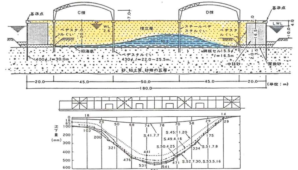
某埋立地の建物例
