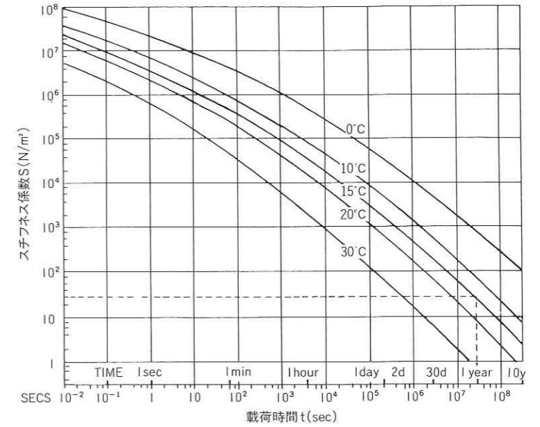
荷重時間とスチフネス係数の関係(グレードB)
