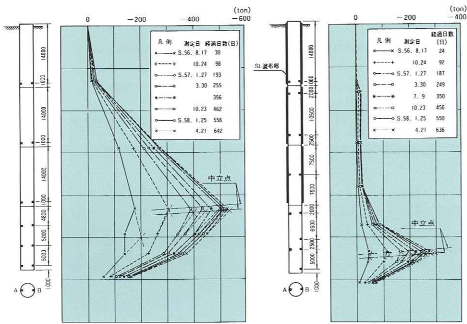
杭体軸力分布図 (SL未塗布杭)
