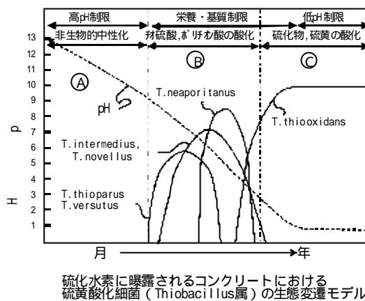
図 - 2 コンクリート腐食に関わる硫黄酸化細菌
