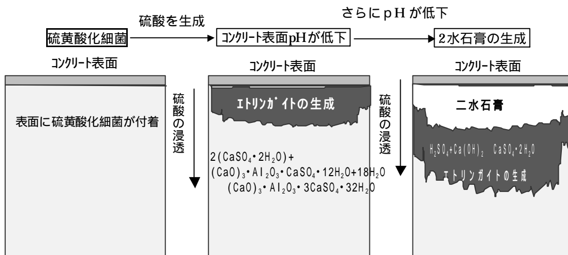
図 - 3 硫酸による劣化進行概念図
