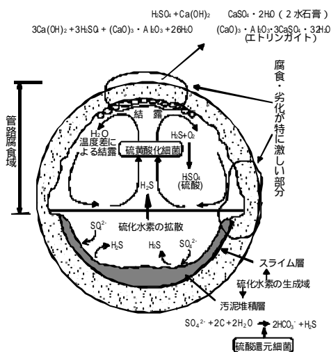
図 - 1 コンクリートの腐食概念図
