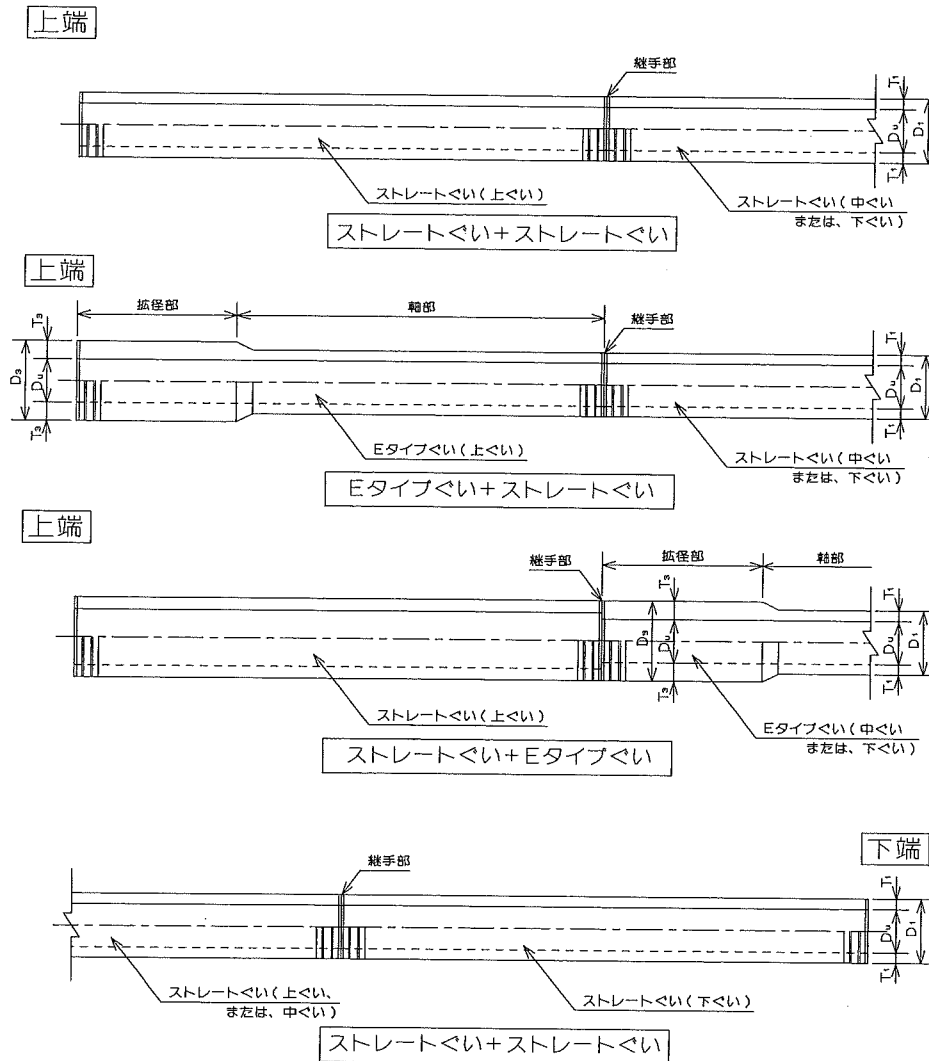
図 I-3-1 標準形状図
