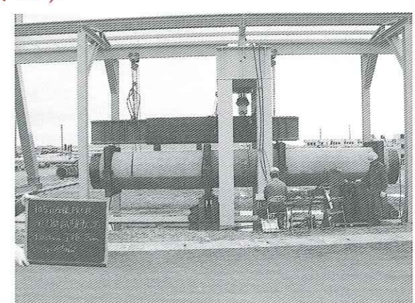
φ1000mm (I種) せん断実験の全景
